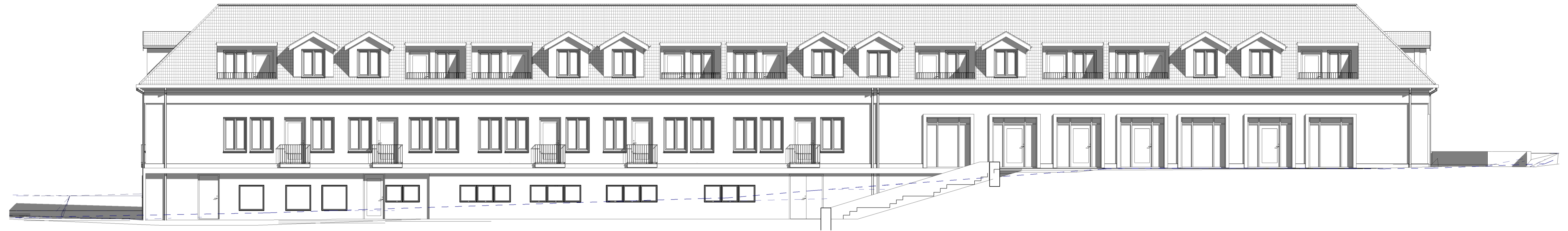
FASAD ÖST 1 : 100
